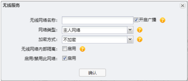
图 2-8 新增无线服务界面
